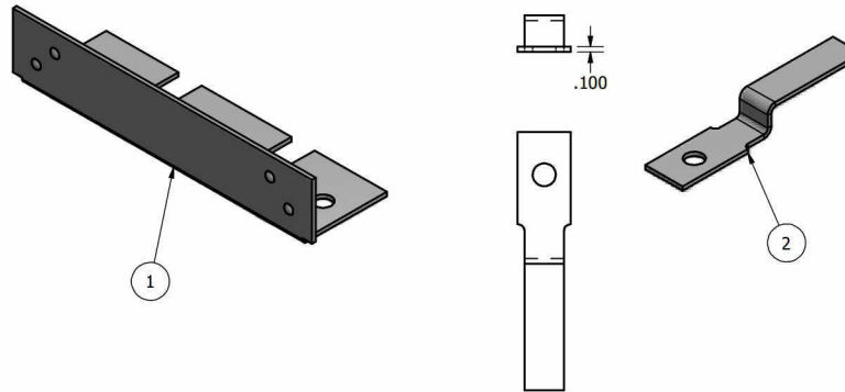
Header Clip (12ga Galvaneal)
