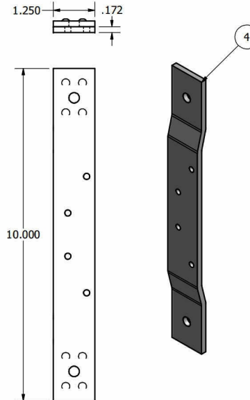
Door Hinge Reinforcement (8ga Galvaneal)
