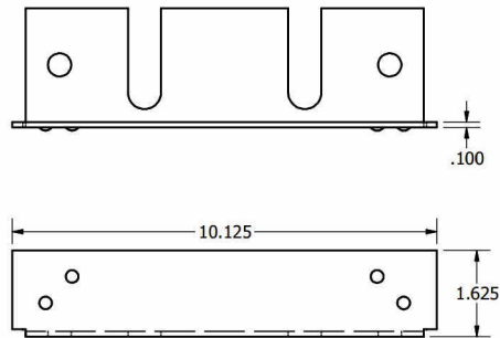
Jamb Clips (12ga Galvaneal)
