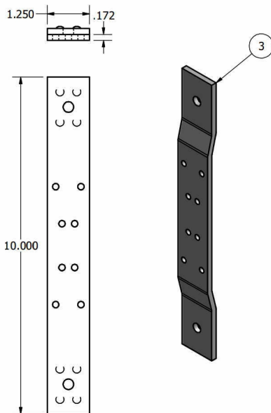
Hinge Jamb Reinforcement (8ga Galvaneal)
